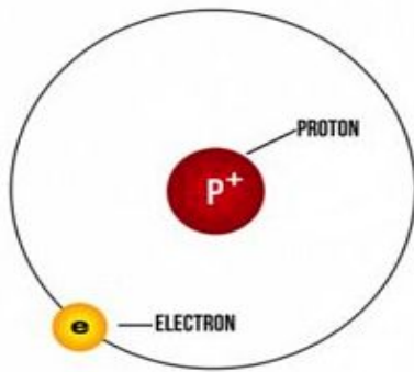
PROTIUM {}^1_1\text{H}
