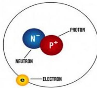
DEUTERIUM {}^2_1\text{H}
